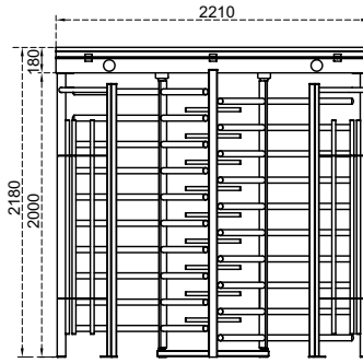
Ölçüler (mm)
