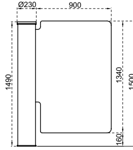
Ölçüler (mm)
